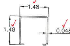
G3RFM147-18-71 1 1/4" STEEL INSERT
